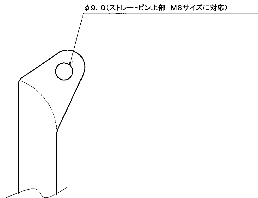
バックステー OarLock側 取付部
