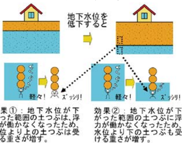
図3 地下水位低下の2重の対策効果
